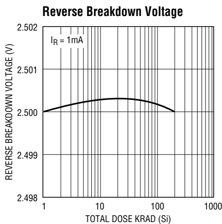
RH1009 G01
