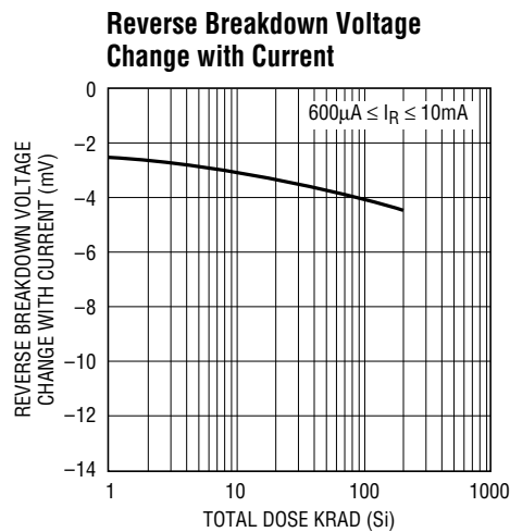
RH1009 G02
